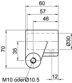
Anschlussstück geschlossen, 1-schalig Connection piece, closed, 1-shell
