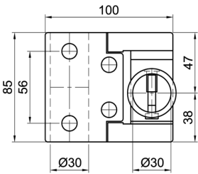
Pendellager 30 x 30, wahlweise 90° oder 180° Swivel bearing 30 x 30 option of 90° or 180°
