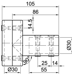
Pendellager 30 x 30, wahlweise 90° oder 180° Swivel bearing 30 x 30 option of 90° or 180°
